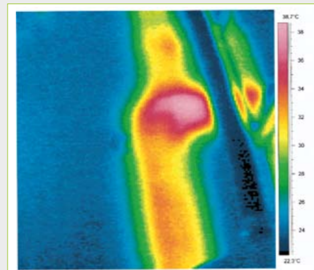
Bild einer Heizungsleckage (Thermografiebild)
